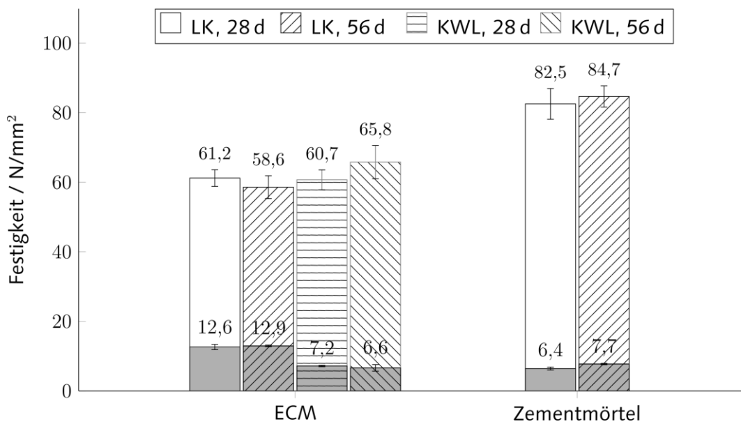
Abb. 2: Druck- (hell) und Biegezugfestigkeit (grau) von Mörteln mit einem Größtkorn von 1,0 mm nach 28 und 56 Tagen unter verschiedenen Klimatischen Bedingungen
