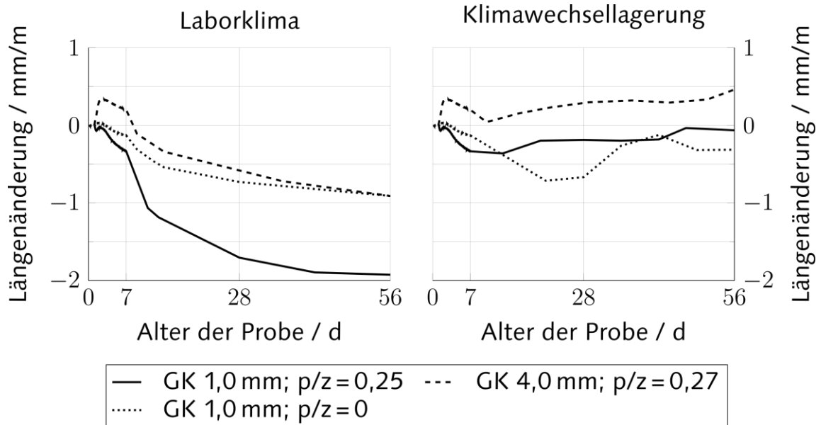
Abb. 1: Gesamtlängenänderung von ECM-Rezepturen mit variierendem Größtkorn im Vergleich zu einem Zementmörtel (gepunktet) unter verschiedenen klimatischen Bedingungen
